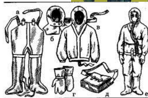
Мал. 305. Легкий захисний костюм Л-1: а — штани з панчохами; б — підшоломиник;
